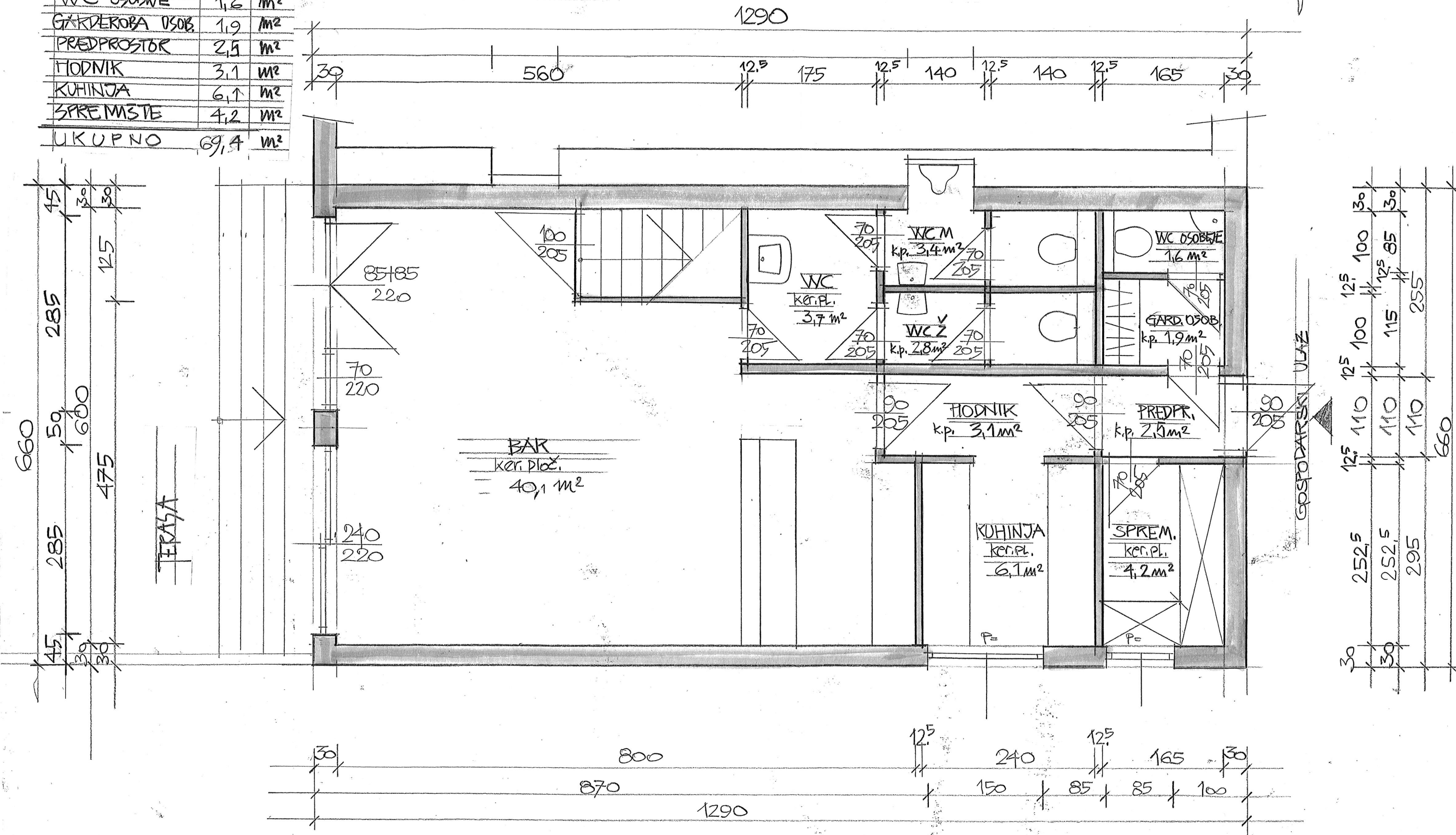
TLOCRT PRIZEMLJA M 1:50
